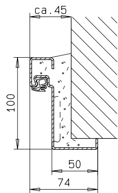
Hauptzarge "ZG/ZNG 68/76"
